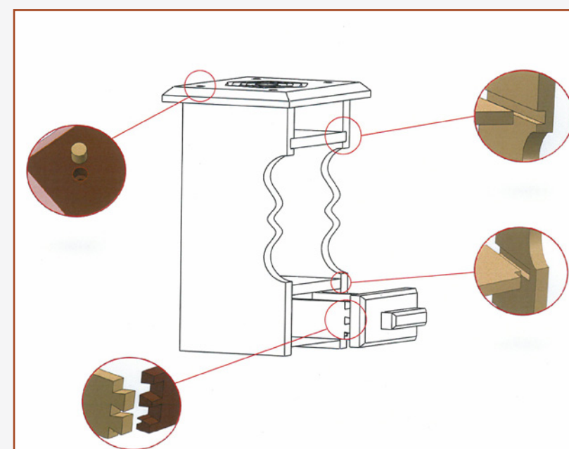
3.18 Déantán a rinneadh i mBlain 2: líníochtaí scartha i léaráid
