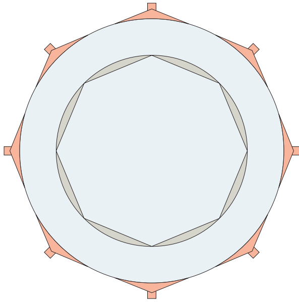
FÍOR 25.5 Balla ochtagánach an chruinneacháin, tógadh boghta cíorlach laistigh de thiús an bhalla agus gearradh taobhanna an ochtagáin amach as an mboghta.
