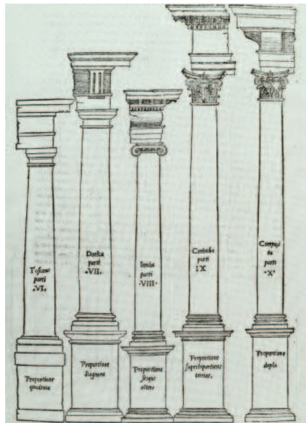
FÍOR 25.8 Oird Chlasaiceacha na hailtireachta
